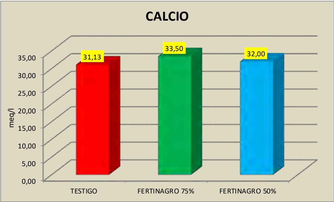
Figura n°33 COMPARATIVA CALCIO EN EL EXTRACTO ACUOSO EN SUELO FINAL EN LOS DIFERENTES TRATAMIENTOS
