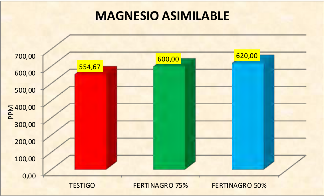
Figura nº37 COMPARATIVA MAGNESIO ASIMILABLE EN SUELO FINAL EN LOS DIFERENTES TRATAMIENTOS
