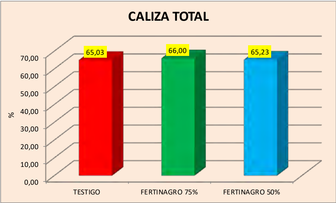
Figura n°45 COMPARATIVA CALIZA TOTAL EN SUELO FINAL EN LOS DIFERENTES TRATAMIENTOS
