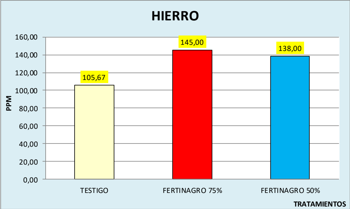
Figura nº24 COMPARATIVA HIERRO EN HOJA DIFERENTES TRATAMIENTOS
