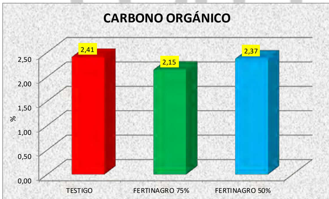
Figura nº40 COMPARATIVA CARBONO ORGÁNICO EN SUELO FINAL EN LOS DIFERENTES TRATAMIENTOS
