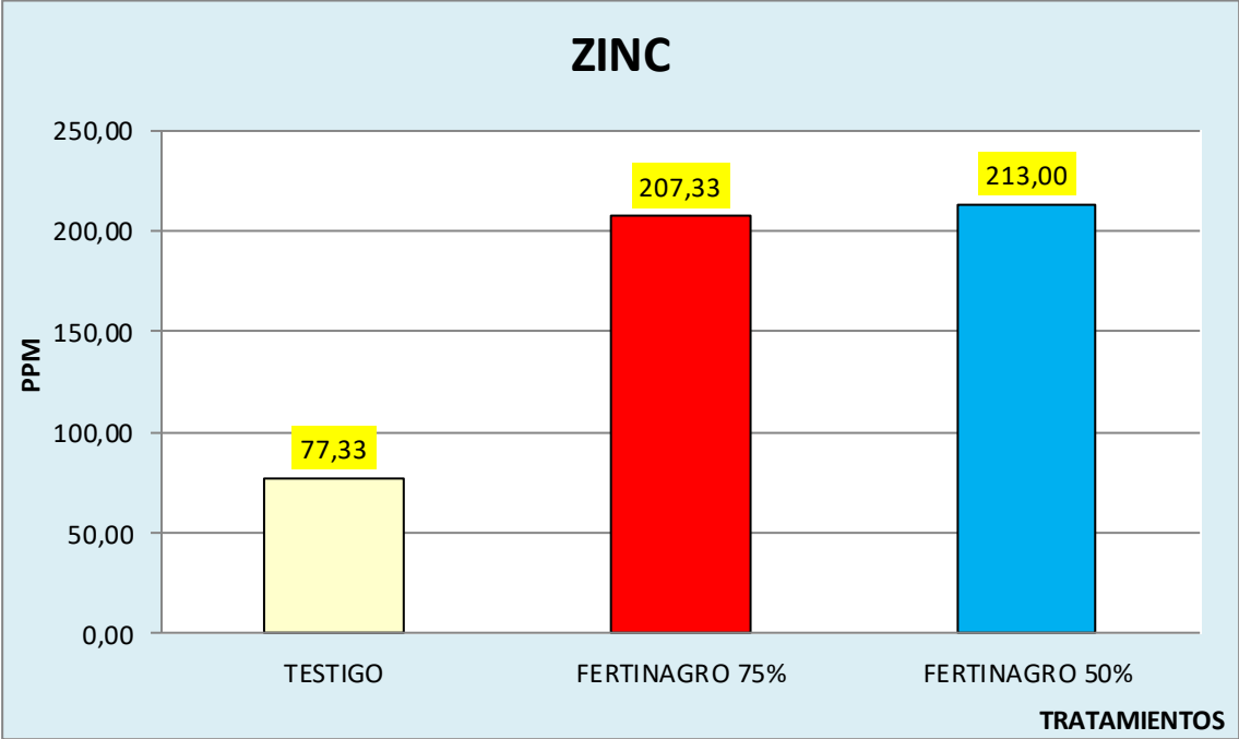
Figura nº25 COMPARATIVA ZINC EN HOJA DIFERENTES TRATAMIENTOS
