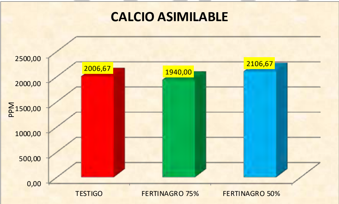
Figura nº38 COMPARATIVA CALCIO ASIMILABLE EN SUELO FINAL EN LOS DIFERENTES TRATAMIENTOS
