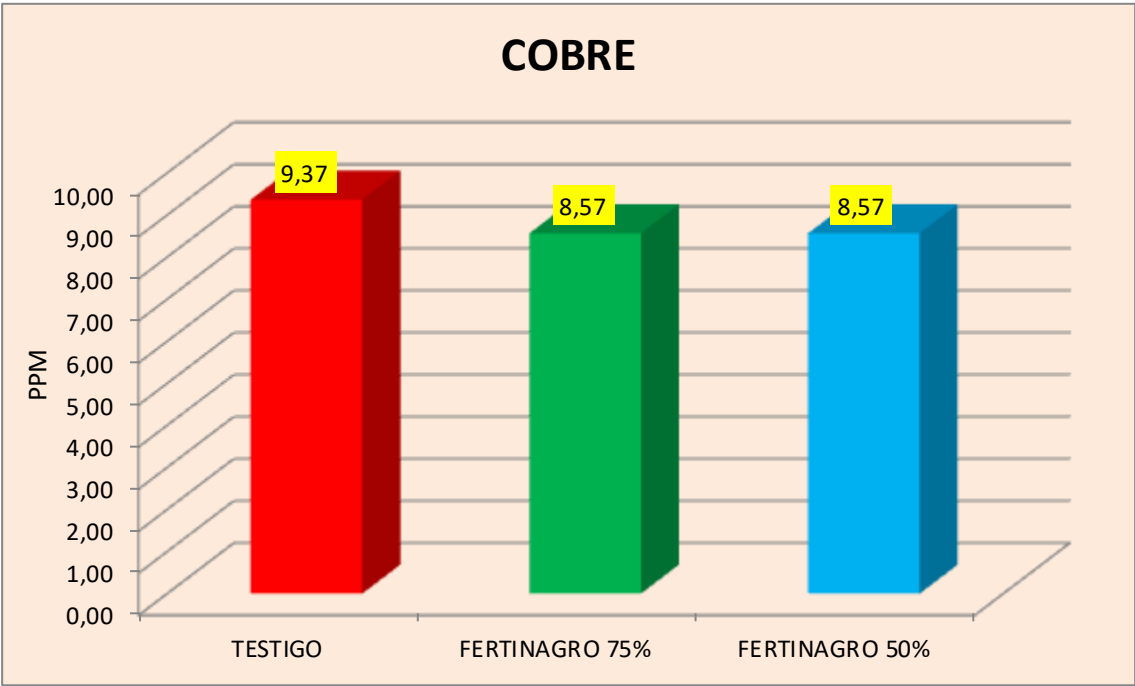
Figura nº43 COMPARATIVA COBRE EN SUELO FINAL EN LOS DIFERENTES TRATAMIENTOS
