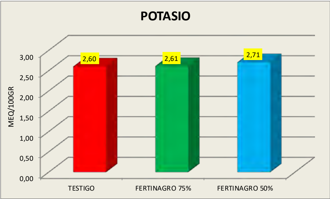
Figura n°49 COMPARATIVA POTASIO DE CAMBIO EN SUELO FINAL EN LOS DIFERENTES TRATAMIENTOS
