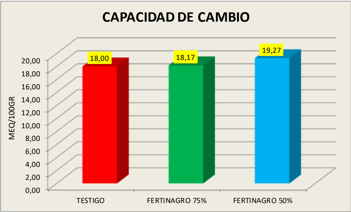
Figura n°51 COMPARATIVA CAPACIDAD DE CAMBIO CATIÓNICO EN SUELO FINAL EN LOS DIFERENTES TRATAMIENTOS
