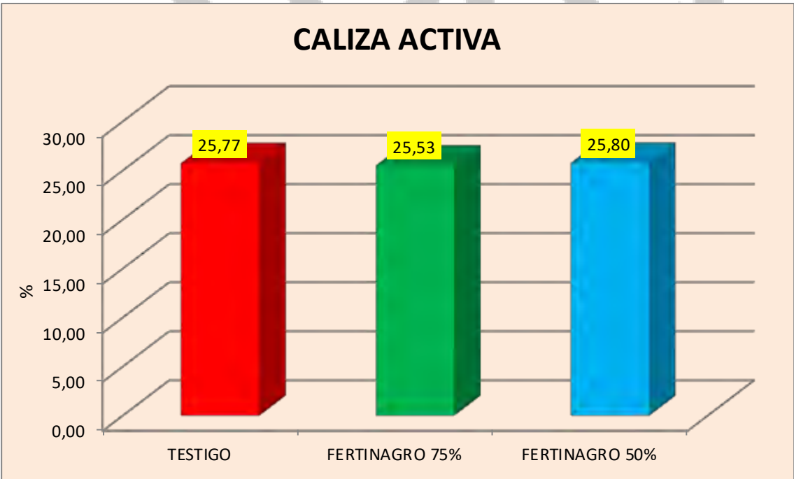
Figura n°46 COMPARATIVA CALIZA ACTIVA EN SUELO FINAL EN LOS DIFERENTES TRATAMIENTOS
