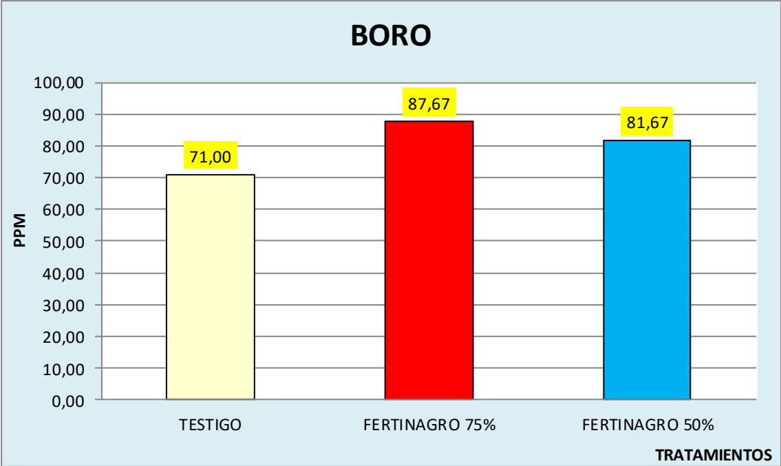
Figura nº22 COMPARATIVA BORO EN HOJA DIFERENTES TRATAMIENTOS
