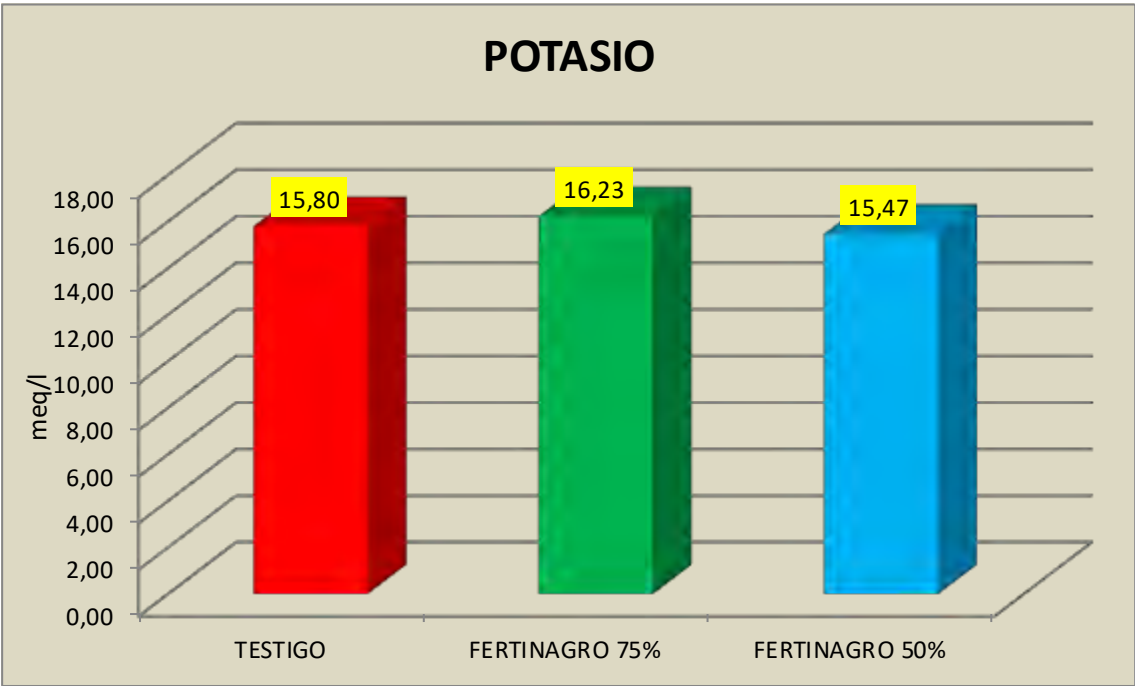
Figura n°32 COMPARATIVA POTASIO EN EL EXTRACTO ACUOSO EN SUELO FINAL EN LOS DIFERENTES TRATAMIENTOS
