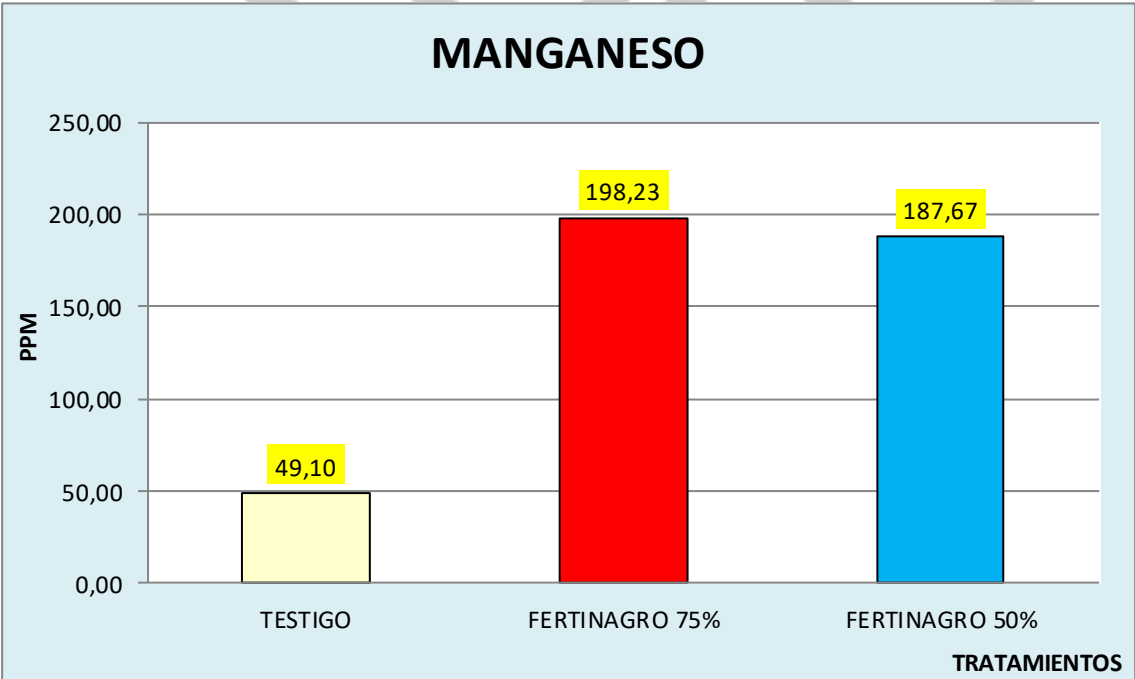
Figura nº23 COMPARATIVA MANGANESO EN HOJA DIFERENTES TRATAMIENTOS
