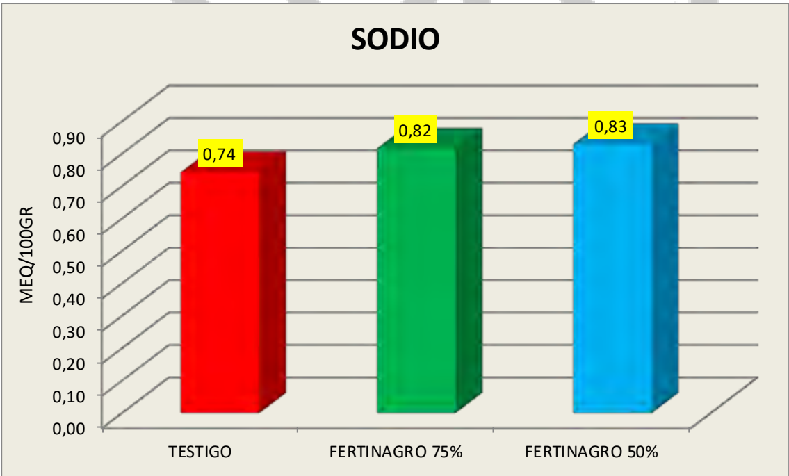
Figura n°50 COMPARATIVA SODIO DE CAMBIO EN SUELO FINAL EN LOS DIFERENTES TRATAMIENTOS
