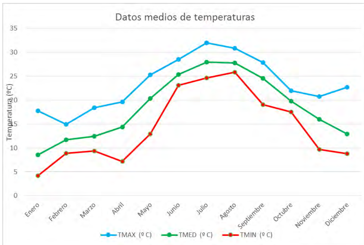
Gráfica 1: Temperaturas medias máxima, media y mínima durante el año 2022. Fuente: Estación AL 52-SIAM-IMIDA.
