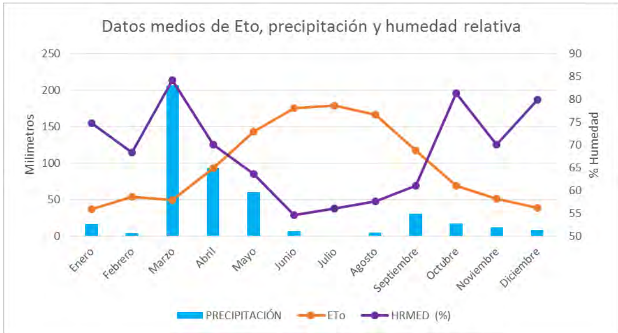
Gráfica 2: Precipitación y evapotranspiración durante el año 2022. Fuente: Estación AL 52-SIAM-IMIDA.
